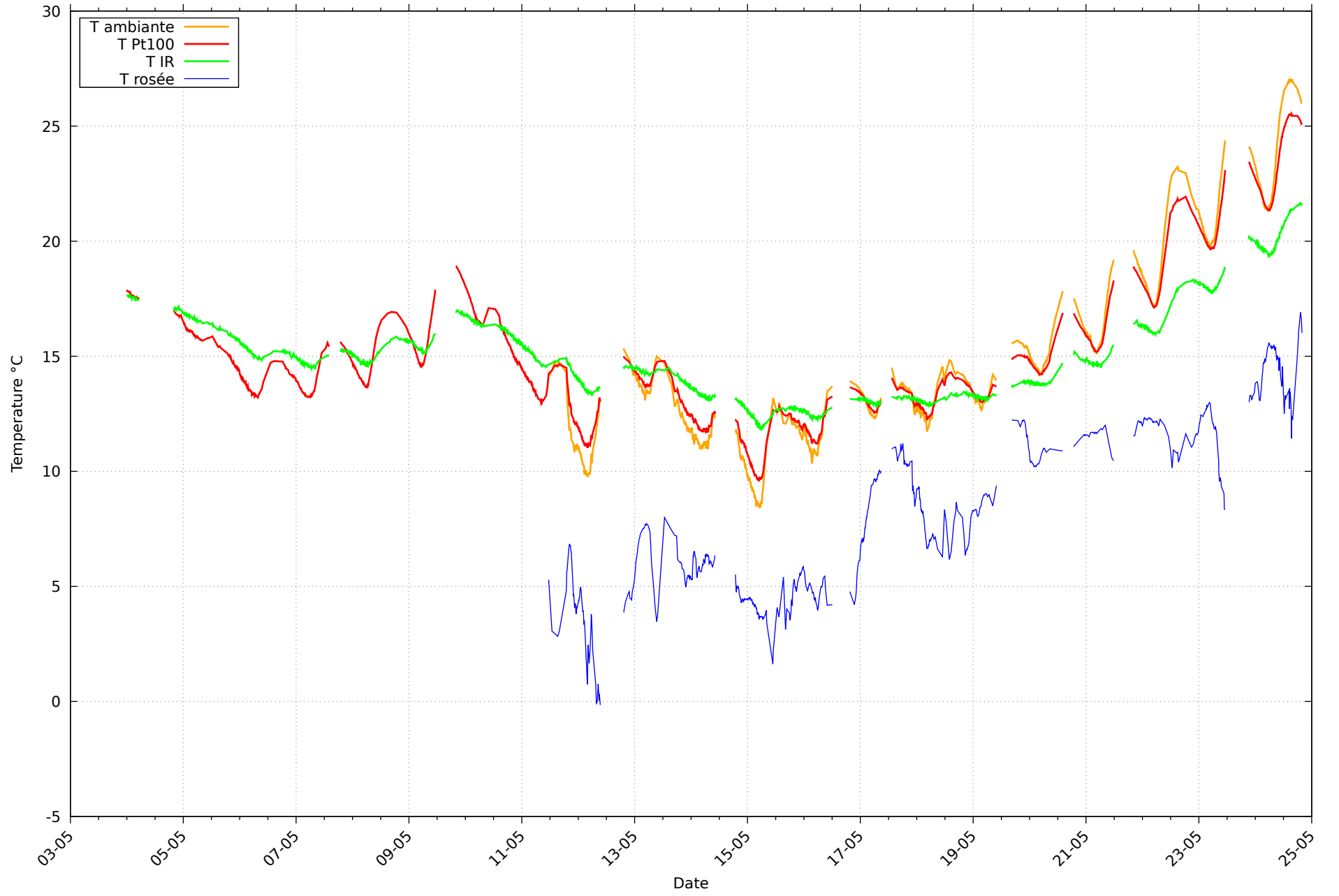
Température et rosée au 24/05/2026 pour RHT10
