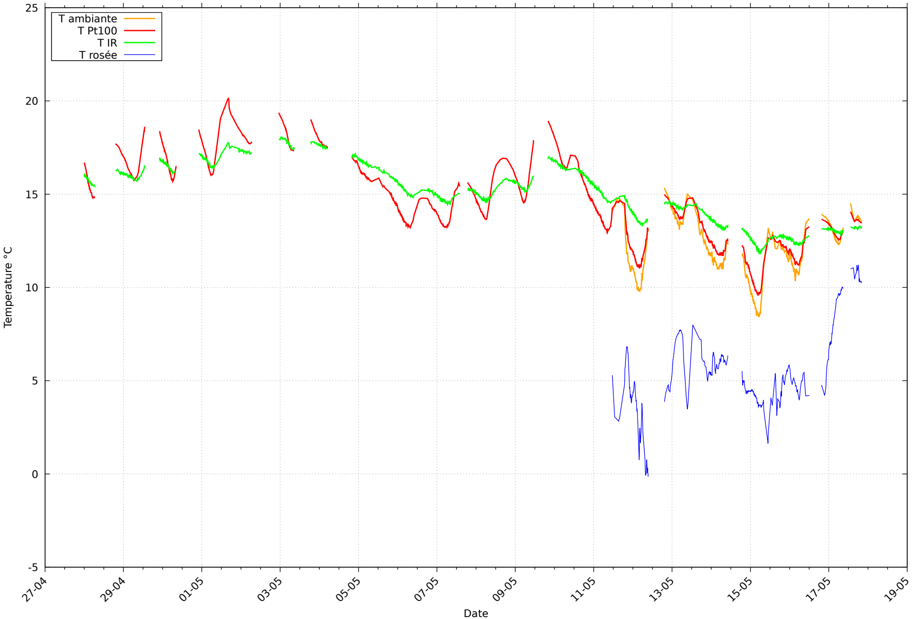
Température et rosée au 17/05/2026 pour RHT10
