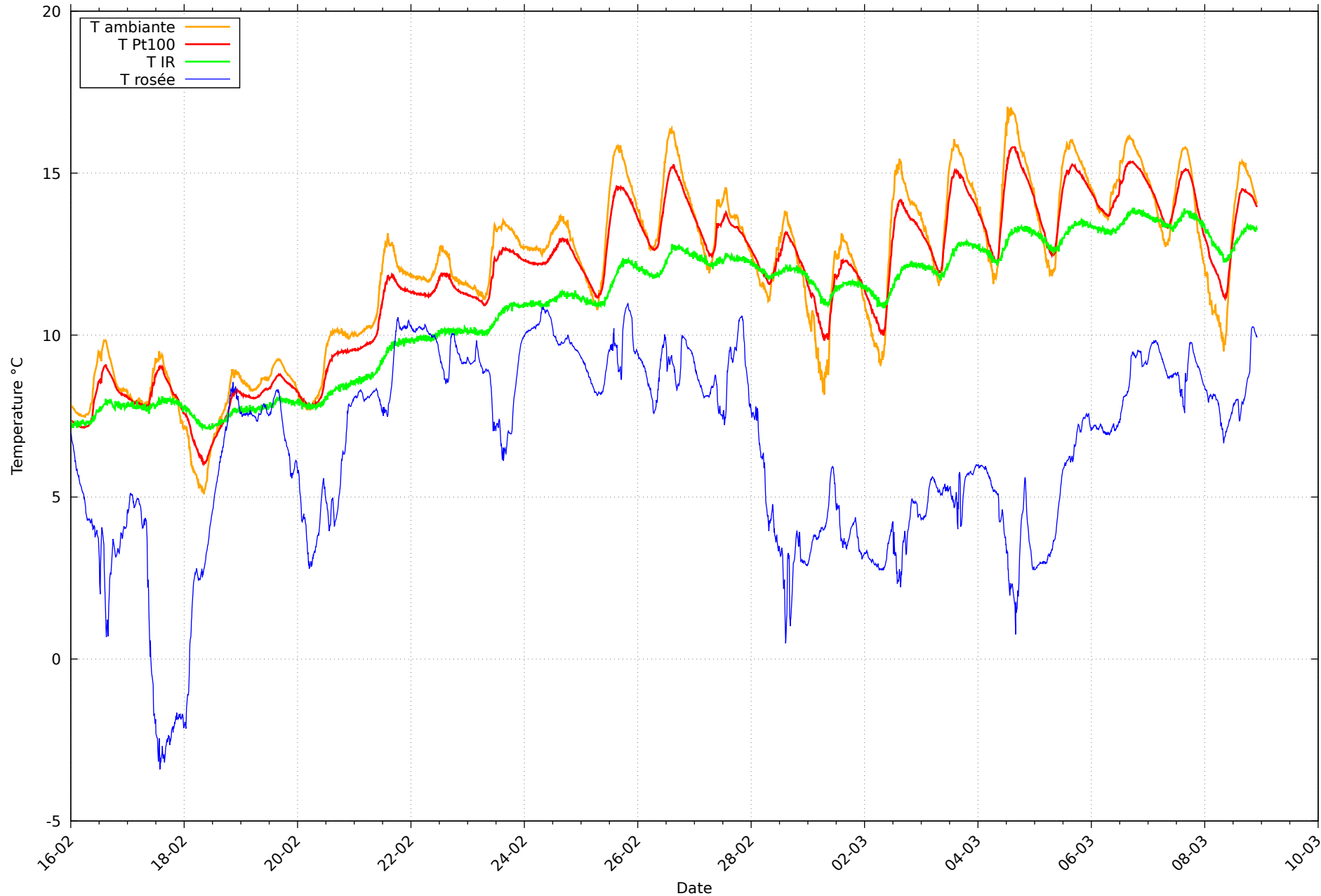
Température et rosée au 08/03/2026 pour RHT10
