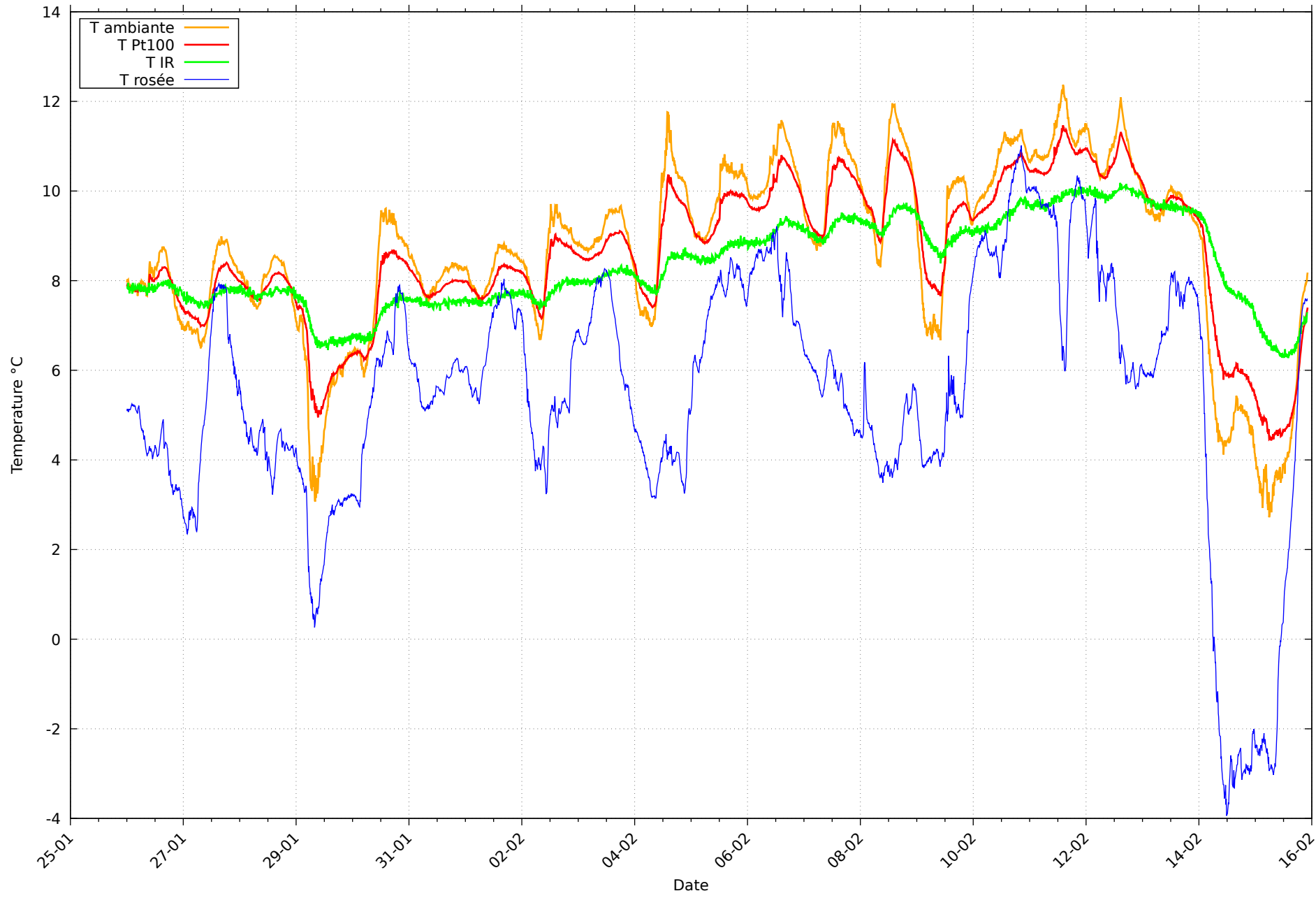
Température et rosée au 15/02/2026 pour RHT10
