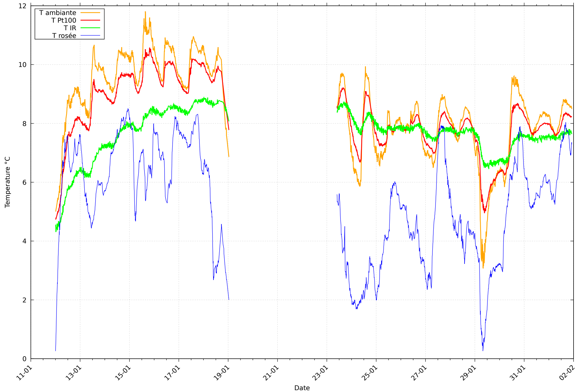
Température et rosée au 01/02/2026 pour RHT10
