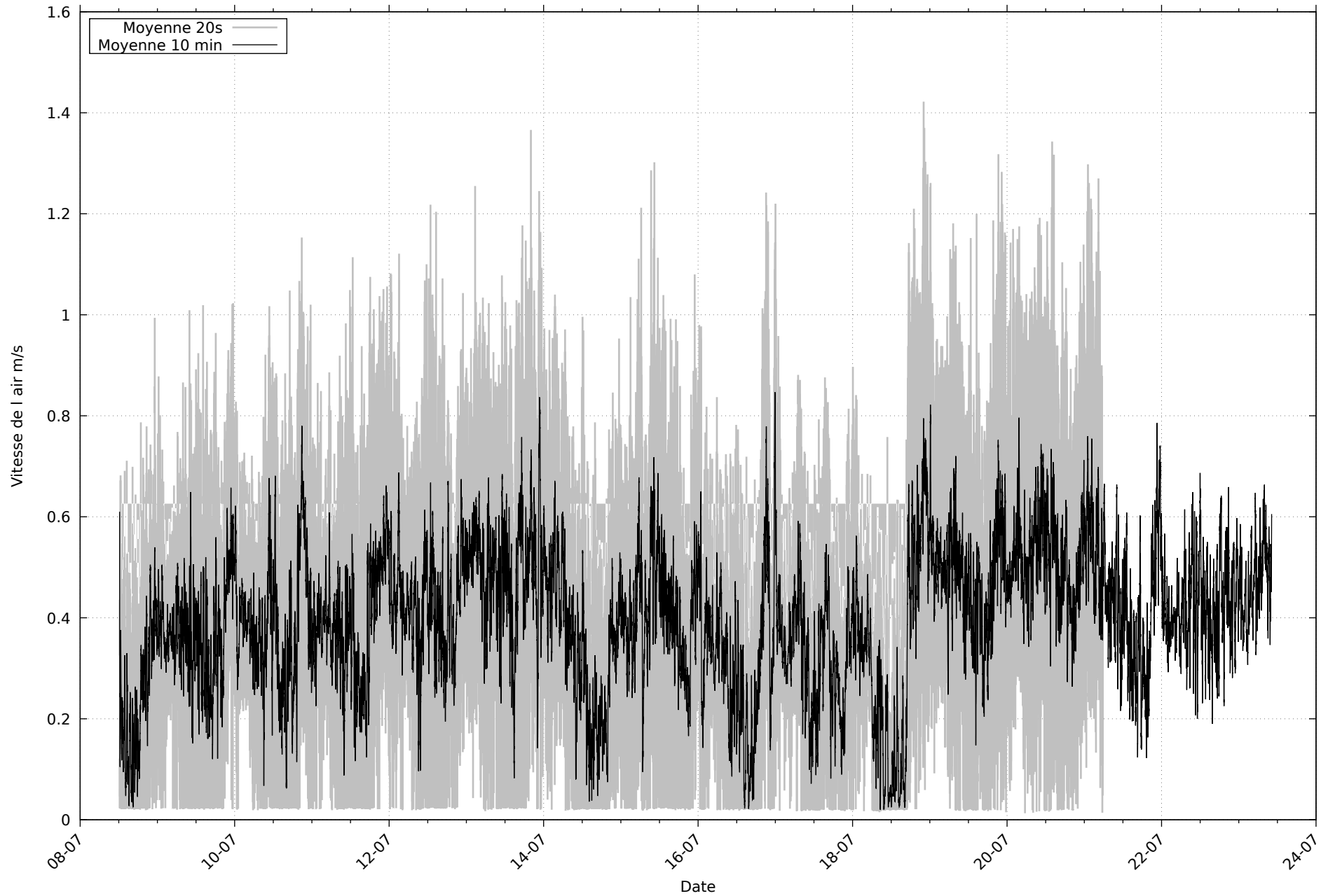
Déplacement d'air au niveau 3 au 26/07/2026
