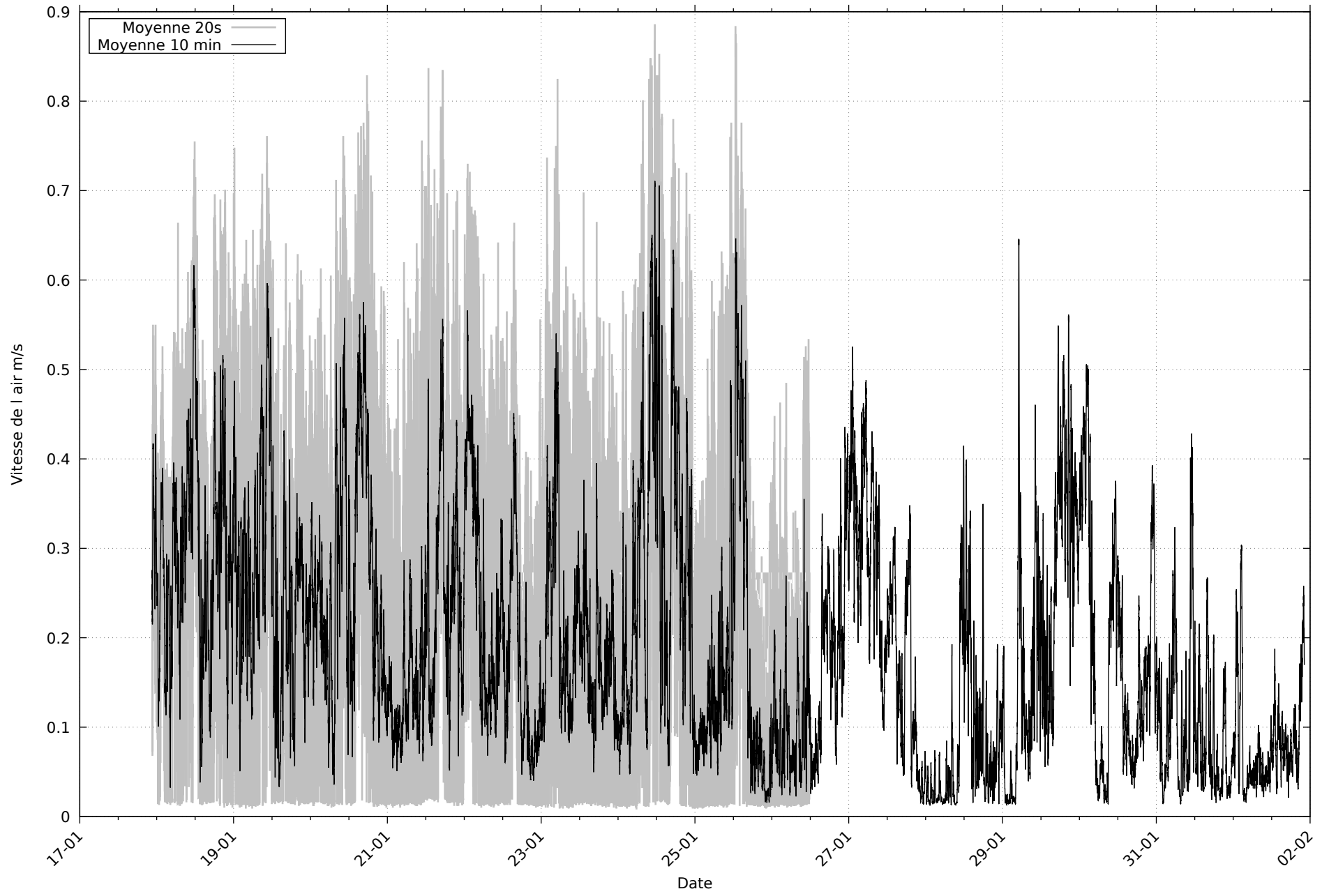
Déplacement d'air au niveau 3 au 01/02/2026
